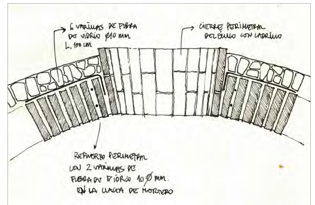
Detalle de óculo en el pozo 11
