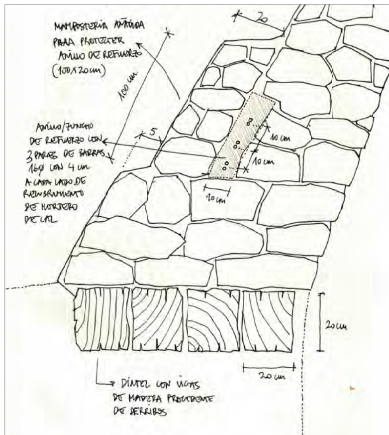
Detalle de arranque de la escalera en acceso sur del pozo 11
