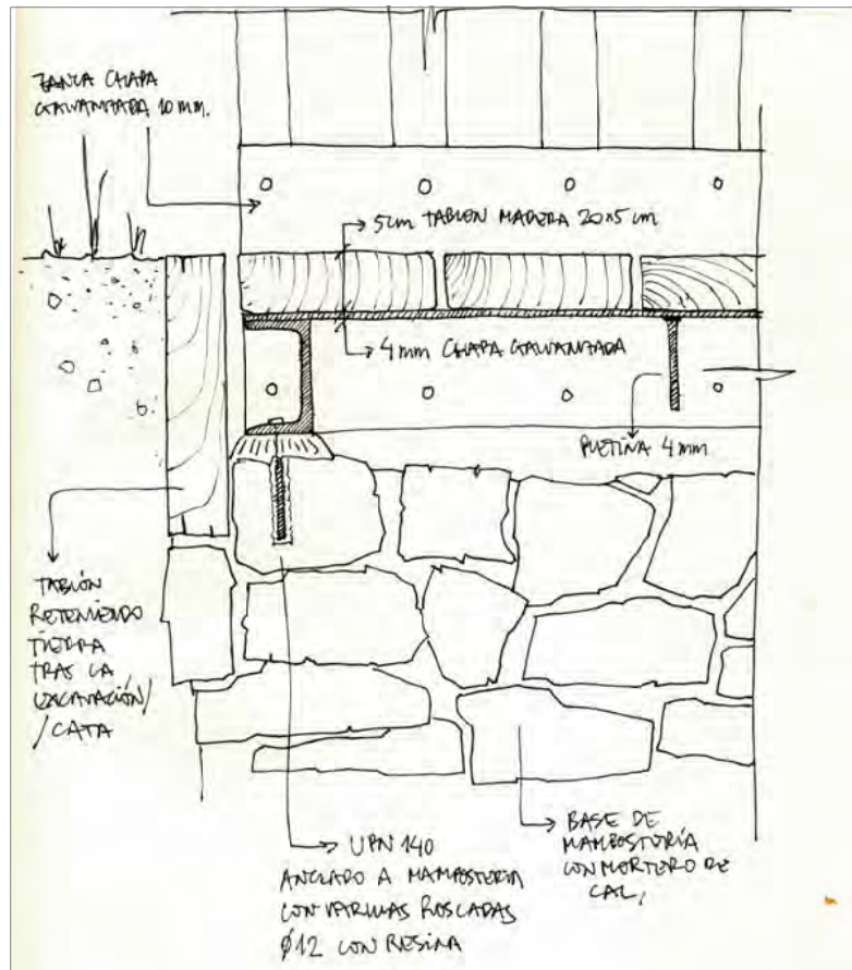
Detalle de arranque de la escalera en acceso sur del pozo 11
