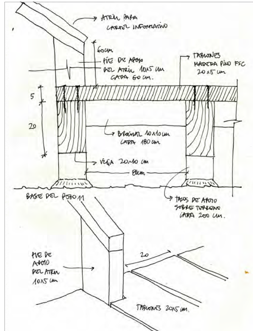
Detalle de plataforma de madera y atril en la base del pozo 11
