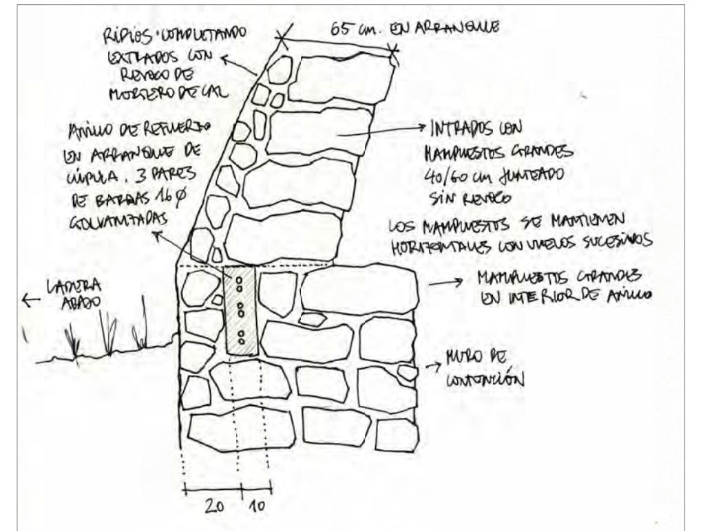
Detalle de encuentro entre el muro de contención y la cúpula del pozo 13
